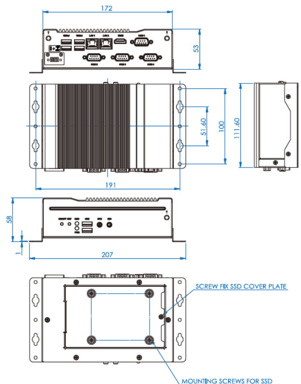
外形寸法図
