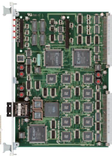
VMEバス用 シェアードメモリボード Advme1522A VxWorks
