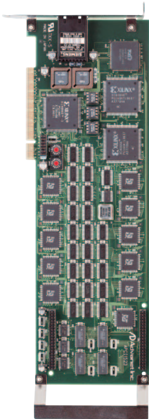
PCIバス用 シェアードメモリボード Adpci1523A VxWorks win3x winNT
