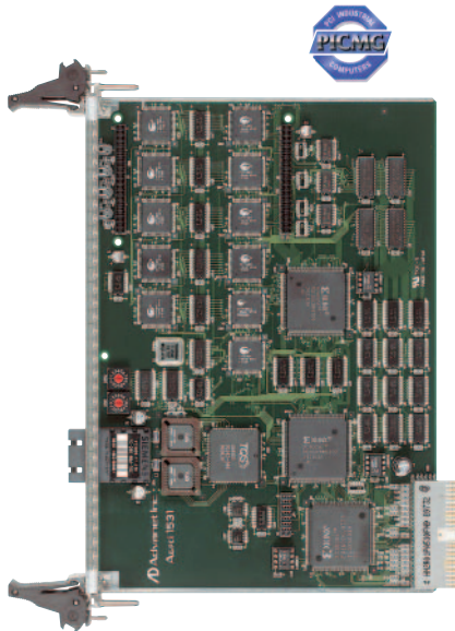
コンパクトPCI用 シェアードメモリボード Agpci1531A VxWorks win3x winNT
